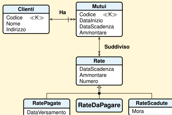
Figura 4.1: Schema concettuale Mutui, Esercizio 2.6
