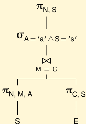
(a) Albero iniziale
