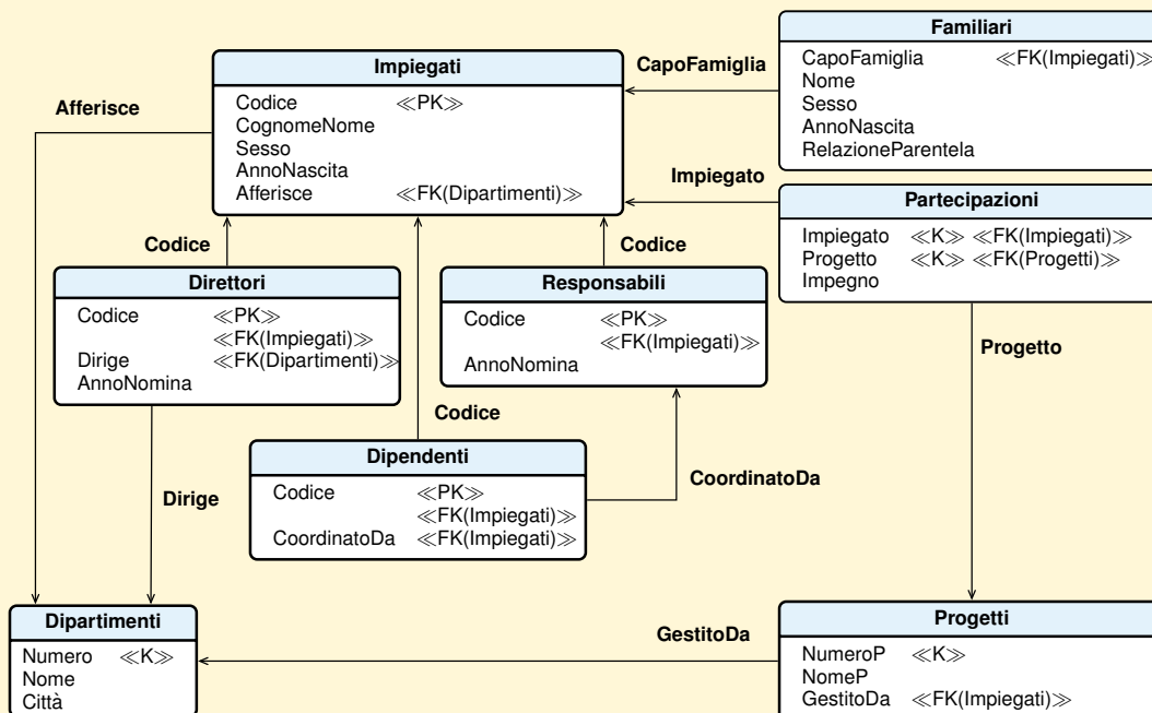
Figura 4.4: Gestione di dati aziendali: progetto relazionale
