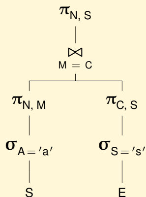
(b) Albero riscritto
