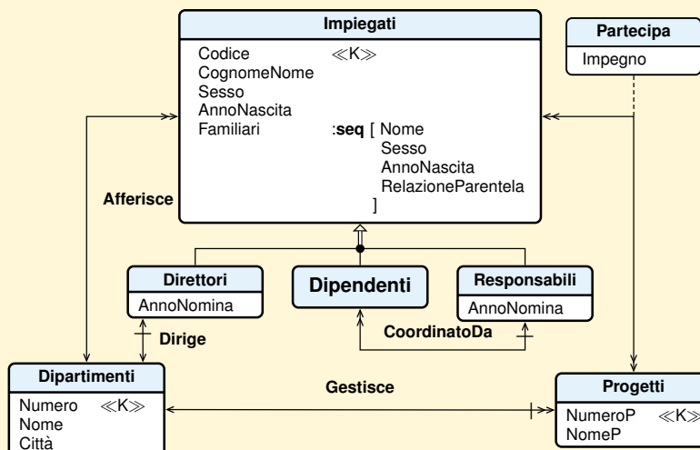
Figura 4.3: Schema concettuale Azienda, Esercizio 2.8
